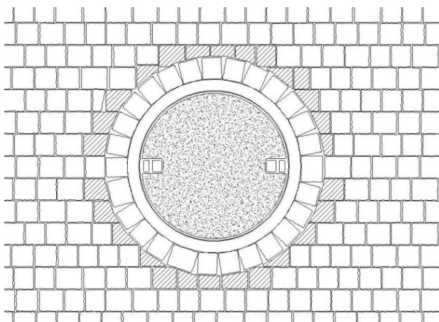
Mögliches Verlegebild bei Schachtanschlüssen. Schraffierte Steine zeigen die zugeschnittenen Passteine an.
