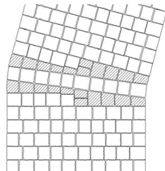
Mögliches Verlegebild bei Wechsel der Verlegrichtung mit FRIEDA® Pflastersteinen. Schraffierte Steine zeigen die zugeschnittenen Passteine an.
