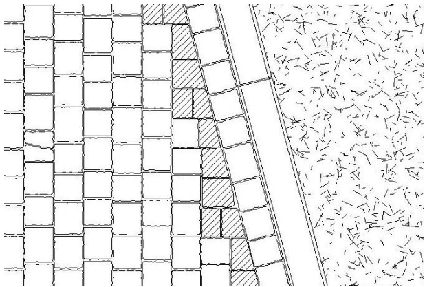
Mögliches Verlegebild beim Anschluss von schräg verlaufenden Abschlüssen. Schraffierte Steine zeigen die zugeschnittenen Passteine an.
