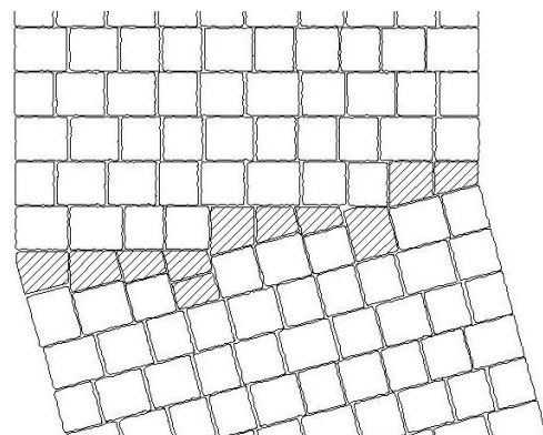
Mögliches Verlegebild bei Wechsel der Verlegrichtung mit FRIEDA® Pflastersteinen. Schraffierte Steine zeigen die zugeschnittenen Passteine an.
