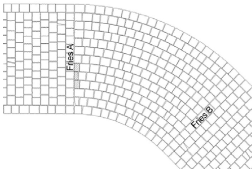
Mögliches Verlegebild bei Wechsel der Verlegrichtung mit FRIEDA® Pflastersteinen. Schraffierte Steine zeigen die zugeschnittenen Passteine an.
